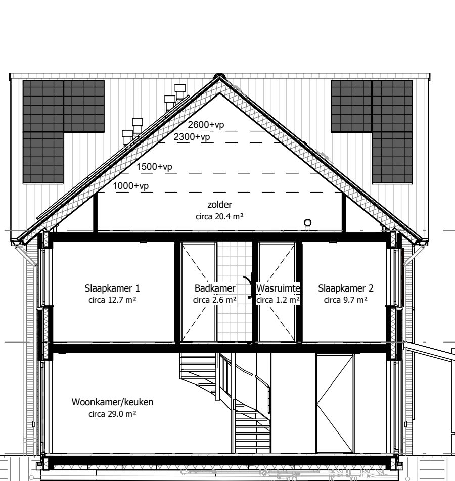
Type: R-Asp Bouwnummer 04 Doorsnede A-A schaal 1:100
