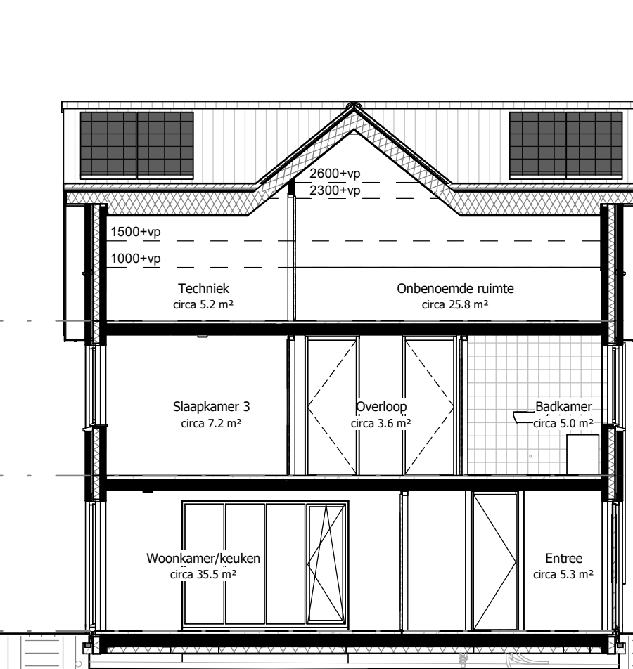
Type: H-B Bouwnummer 06 Doorsnede B-B schaal 1:100
